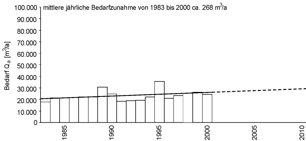
Abb. 12: Bedarf Q_a von ST Bergfreiheit von 1983 bis 2000 und erwarteter Bedarfsverlauf bis 2010
