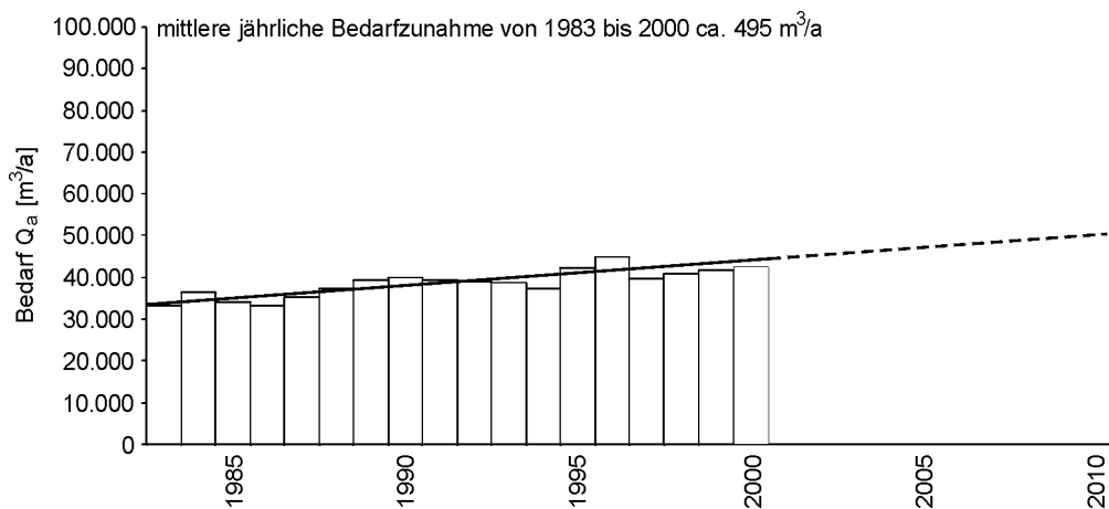
Abb. 13: Bedarf Q_a von ST Braunau von 1983 bis 2000 und erwarteter Bedarfsverlauf bis 2010
