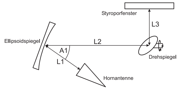
Abbildung D.1: Maße der Wasserdampf Quasioptik.
