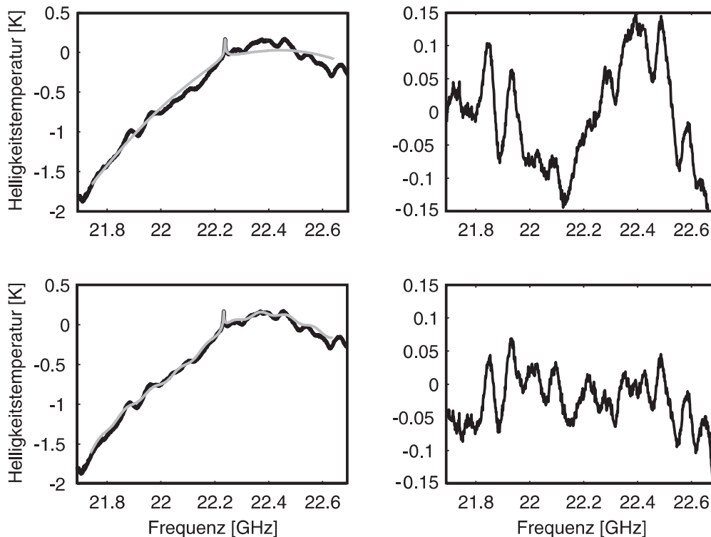
Abbildung 6.7: Oben: Links das Spektrum und Vorwärtsspektrum (grau) einer Wasserdampfmessung ohne angepaßte Stehwellen; Rechts das Residuum bestehend aus Spektrum abzüglich dem Vorwärtsspektrum. Die Effekte der Stehwellen liegen in der gleichen Größenordnung wie die Stärke der zentralen Wasserdampflinie von etwa 0,15 K. Unten: Links Spektrum und Vorwärtsspektrum (grau) mit den zwei angepaßten Stehwellen, Rechts das zugehörige Residuum. Es zeigt sich, daß trotz der Anpassung noch immer deutlich Stehwelleneffekte erkennbar sind; im Gegensatz zu oben-rechts sind sie jetzt jedoch nicht mehr in der Größenordnung der beobachteten Wasserdampflinie (Daten vom 25. November 1999).
