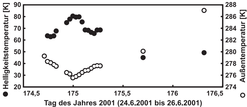
Abbildung 8.4: Die mittleren Helligkeitstemperaturen der einzelnen Messungen (schwarze Kreise) sowie die vor dem Labor gemessenen Außentemperaturen (weiße Kreise).
