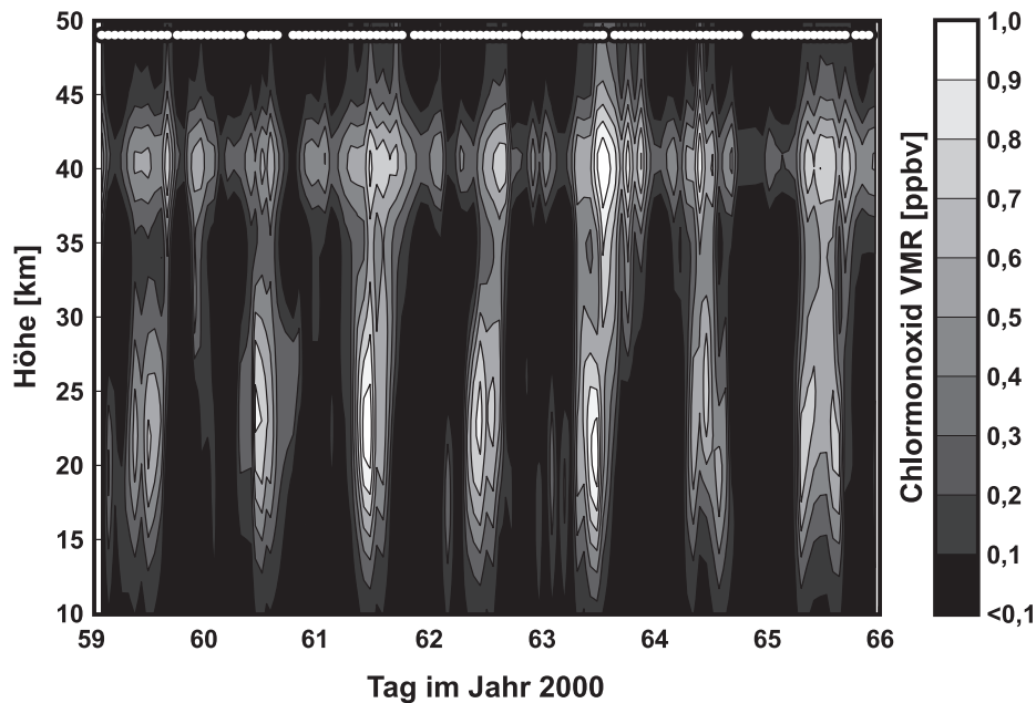
Abbildung 7.13: Die Konzentration von Chlormonoxid der Tage vom 29. Februar (Tag 59) bis zum 6. März 2000 (Tag 65) für die Höhen von 10 bis 50km. Im Beobachtungszeitraum fanden insgesamt 115 Messungen statt (markiert durch weiße Punkt am Oberrand der Grafik). Sie wurden jeweils mit einer passenden mittleren Nachtmessung als »Messung Minus Nacht« Spektrum verrechnet und anschließend invertiert.
