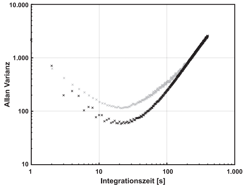
Abbildung 6.11: Die Mittlere Allan Varianz der Spektrometerkanäle des Wasserdampf Radiometers mit Blick auf die kalte Last (schwarz) und die warme Last (grau). Das Minimum der Varianz zeigt die optimale Integrationszeit. Links dieses Punktes wirken sich kurzzeitige Schwankungen durch Rauschen, rechts die langfristige Drift der Verstärker störend aus.
