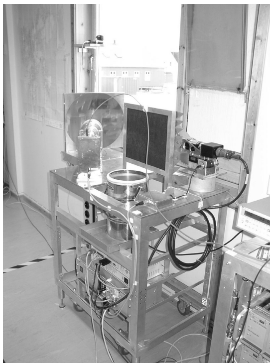
Abbildung 6.8: Das Wasserdampf Radiometer im NDSC Observatorium in Ny-Ålesund. Über das Empfangshorn mit der Frontendelektronik hinweg blickt man direkt in den großen elliptischen Fokussierspiegel. Auf der Grundplatte rechts, auf einem Absatz befindet sich der Weglängenmodulator mit dem Motor für den Drehspiegel, der bei dieser Perspektive durch die warme Last verdeckt ist. Der im Bild erkennbare Behälter mit dem Stickstoff wird zur Kalibration unter den Drehspiegel geschoben. Im oberen Bereich des Styroporfensters erkennt man die für Referenzstrahlungsmessungen benötigte Plexiglasplatte. Im Rack unterhalb der Grundplatte sind die Versorgungs-, Steuer- und Schalteinrichtungen des Radiometers untergebracht. Die Zwischenfrequenzkette mit dem Spektrometer befindet sich im rechts benachbarten Rack des Ozon Radiometers.
