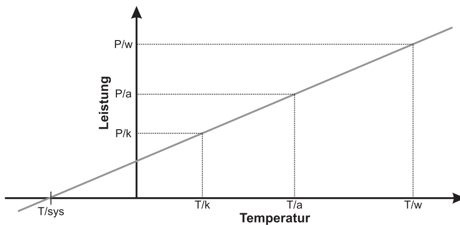
Abbildung 4.1: Schema für die Kalibration der Strahlungsleistung mittels der Totalpower Methode. T/k und T/w sind die Temperaturen der kalten und warmen Kalibrationslast mit den gemessenen Leistungen P/k und P/w . Aus der gemessenen atmosphärischen Strahlungsleistung P/a kann die Temperatur der Atmosphäre T/a bestimmt werden. Mittels Gleichung (4.5), der Y-Faktor Methode, kann aus den Messungen der warmen und der kalten Last auch die Systemrauschtemperatur T/\text{sys} bestimmt.
