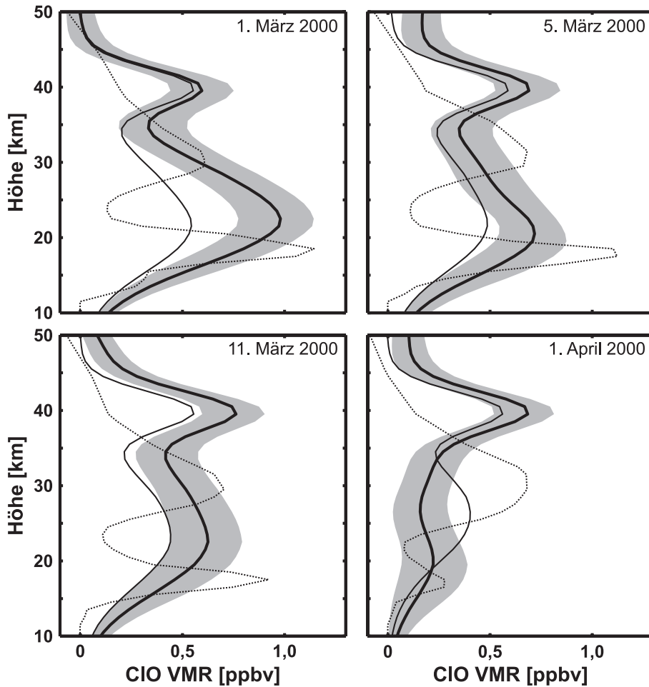
Abbildung 7.10: Ein detaillierter Vergleich von vier beispielhaft ausgewählten Messungen des RAM mit dem Modell SLIMCAT. Die RAM Messungen sind als dicke Linie mit Fehlerbereichen dargestellt; SLIMCAT in originaler Höhenauflösung wird als Punktlinie sowie in RAM Höhenauflösung als durchgezogene Linie dargestellt.
