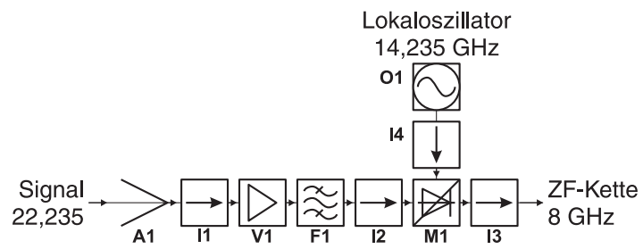
Abbildung D.2: Der elektronische Teil des Wasserdampf Radiometers.
