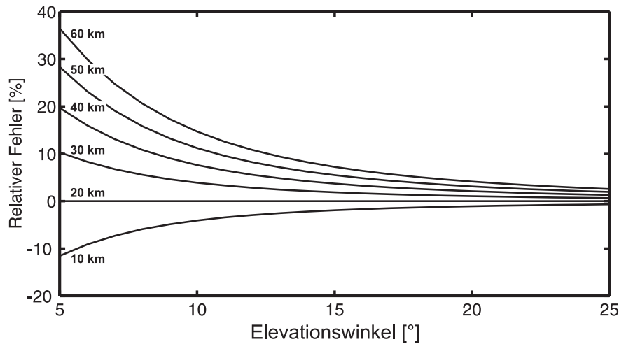
Abbildung 4.4: Der relative Fehler bei der Umrechnung eines Spektrums auf Zenit Beobachtungsgeometrie. Die Referenzhöhe h für den Airmass-Faktor beträgt hier 20 km.
