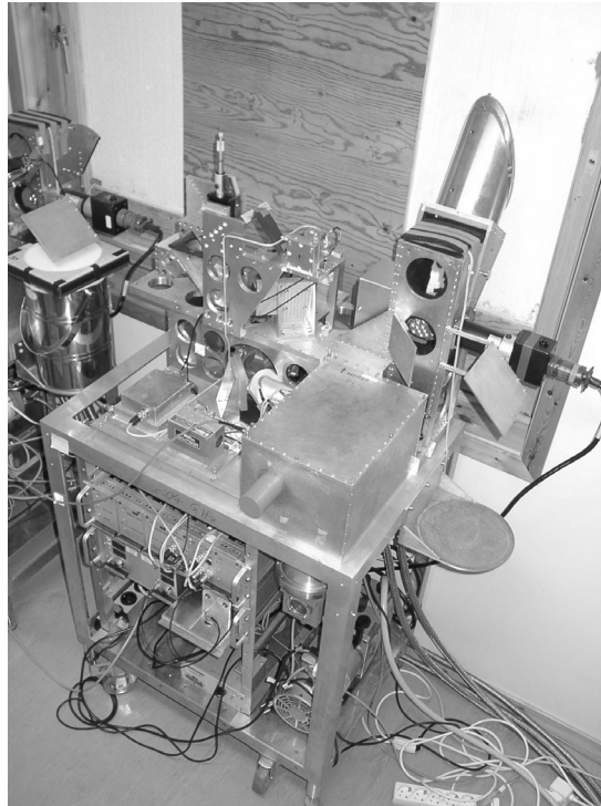
Abbildung 6.4: Das Chlormonoxid Radiometer im NDSC Observatorium in Ny-Ålesund. Auf der Grundplatte befindet sich die Quasioptik aus Spiegeln, Polarisationsgittern und Interferometern; links erkennt man die Mikrometerschraube zur Anpassung des Seitenbandfilters, in der Mitte befindet sich der Lokaloszillator und rechts im Turm der drehbare Spiegel. Der rechteckige Block vorne-rechts ist das Druckgehäuse mit Mischer und Verstärker, darunter befindet sich die Kühlpumpe. Im Rack unterhalb der Grundplatte sind die Versorgungs-, Steuer- und Schalteinrichtungen des Radiometers untergebracht. Die Zwischenfrequenzkette mit dem Spektrometer befindet sich im linken, benachbarten Rack des Ozon Radiometers.
