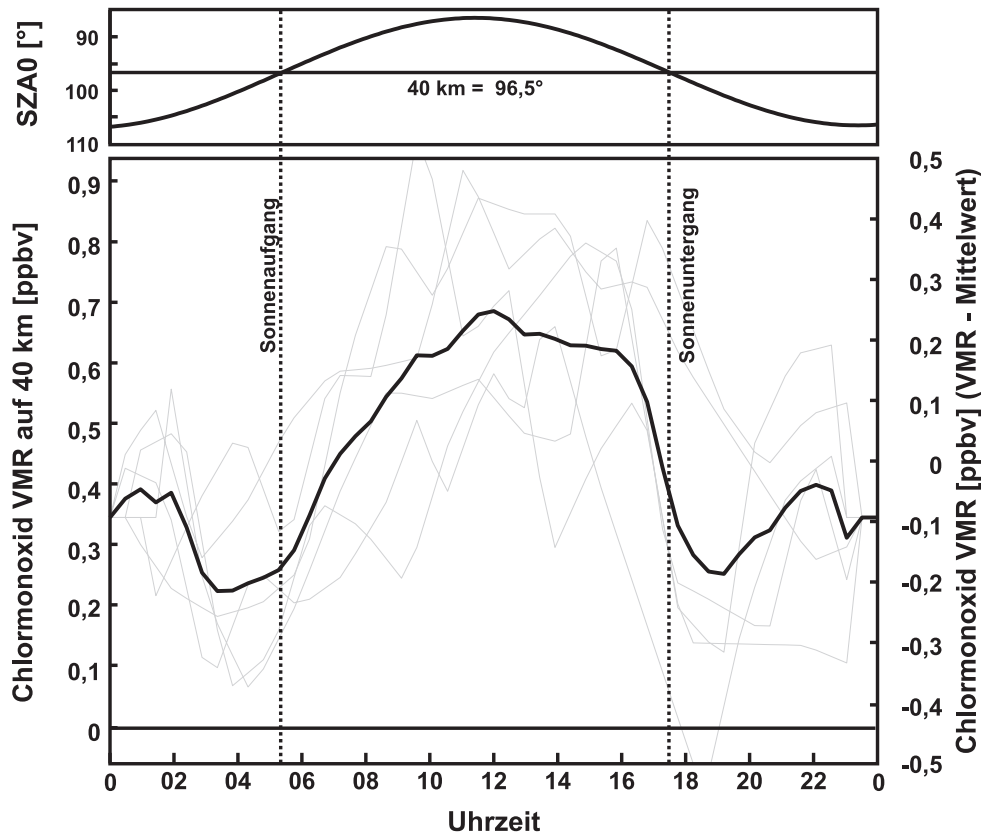
Abbildung 7.17: Ein aus sechs Tagen berechneter mittlerer Tagesgang; gemittelt über einen Höhenbereich von 38 bis 42 km. Tag 63 wurden wegen der großen nachmittäglichen Überschwinger nicht in die Mittelung übernommen. Die sechs einzelnen Tage sind als dünne graue Linien unterlegt. Die linke Sekundärachse zeigt das absolute VMR. Zum besseren Vergleich mit Abbildung 7.18 wurde auf der rechten Ordinate zusätzlich die Variation abzüglich des Tagesmittelwertes aufgetragen. Über der Abbildung befindet sich ein Diagramm mit dem Sonnen Zenitwinkel des Tages. Die Zeiten für den Sonnenaufgangs und Sonnenuntergangs sind markiert.
