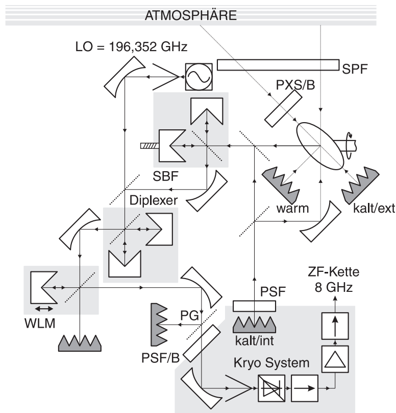
Abbildung 6.2: Eine schematische Darstellung des Chlormonoxidradiometers auf dem aktuellen Stand des Jahres 2001. SPF bezeichnet das Styroporfenster, PXS/B bezeichnet eine Plexiglasplatte die sich unter dem Brewsterwinkel im Referenzstrahl befindet, WLM bezeichnet den Weglängenmodulator und SBF das als Seitenbandfilter verwendete Martin-Puplett-Interferometer. Mit PSF sind die als Ersatz für die Mylarfenster im Januar 1999 eingebauten Polystyrolfenster, wobei das Fenster PSF/B zusätzlich unter dem Brewsterwinkel im Strahlengang steht. Der Polarisationsgitter PG wurde im Januar 2000 zusätzlich eingebaut.
