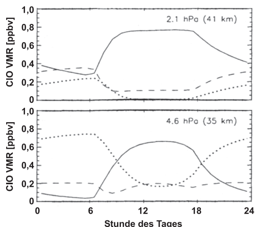
Abbildung 7.19: Eine 0d photochemische Modellrechnung für den Monat Februar nach Ricaud et al. (2000) für 35 und 41 km Höhe. Die durchgezogene Linie entspricht dem Chlormonoxid VMR, die Punktlinie ist \text{ClONO}_2 und die Strichlinie \text{HOCl} . Bei einsetzendem Sonnenlicht würde ein Teil des Tages \text{ClO} durch Photolyse in atomares Chlor umgesetzt werden. Als Folge würde über Mittag die Chlormonoxid Konzentration wieder absinken, so daß sich eine Struktur mit zwei Maxima ausbilden würde.
