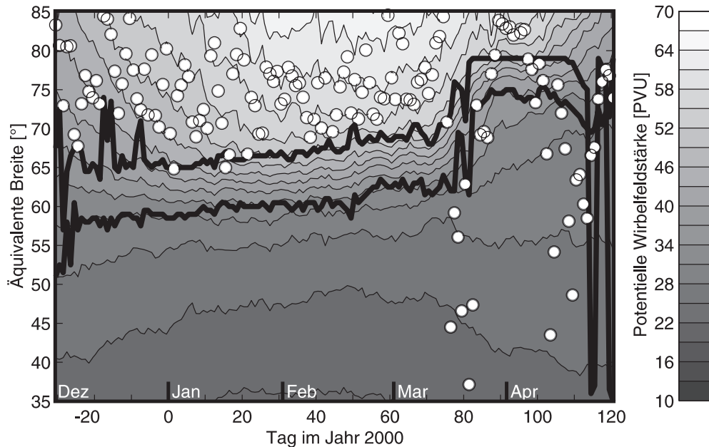
Abbildung 7.3: Der nördliche Polarwirbel für den Winter 1999/2000, dargestellt durch die potentielle Vortizität auf der äquivalenten Breite. Die weißen Punkte entsprechen dem Standort Ny-Ålesund, die dicken Linien sind der innere und äußere Wirbelrand. Von Januar bis Mitte März 2000 war der Wirbel mit einem hohen Gradienten der PV in seinem Randbereich sehr stabil; danach spaltete er sich, um noch bis Mitte April in kleinerer Ausdehnung weiter zu existieren (Berechnet aus Daten des ECMWF).
