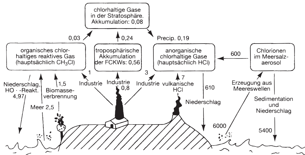
Abbildung 2.3: Der globale Chlorhaushalt, entnommen aus Graedel und Crutzen (1994). Die Einheit für die Flüsse ist 10^{12} g Chlor pro Jahr und galt so bis in die 1990er Jahre – mittlerweile haben sich die Einträge für FCKSWs durch die 1997 im Abkommen von Montreal festgeschriebenen Bemühungen zum Schutz der Ozonschicht vermindert. Man muß bei dieser Abbildung noch anmerken, daß gerade die ozeanischen Flüsse nicht genau bestimmbar und diese Zahlen damit sehr fehlerbehaftet sind. Interessant ist, daß die natürlichen Flüsse in der Troposphäre um mehrere Größenordnungen über den durch Menschen gemachten liegt, wobei die hohe Stabilität der FCKWs hier natürlich die entscheidende Rolle spielt.
