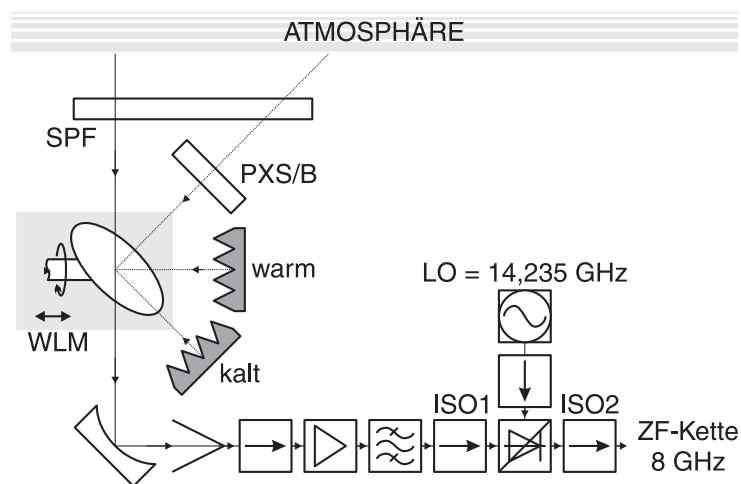
Abbildung 6.5: Eine schematische Darstellung des Wasserdampfradiometers auf dem aktuellen Stand des Jahres 2001. SPF bezeichnet das Styroporfenster, PXS/B bezeichnet eine Plexiglasplatte die sich unter dem Brewsterwinkel im Referenzstrahl befindet. WLM bezeichnet den Weglängenmodulator, auf dem der drehbare Spiegel montiert ist. ISO1 ist der im Frühjahr und ISO2 der im Sommer 1999 nachträglich eingebaute Isolator.
