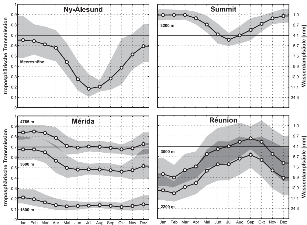
Abbildung 3.4: Modellrechnungen für die Transmissionen der vier Standorte mit ihren verschiedenen Beobachtungshöhen, berechnet jeweils für Zenit Beobachtungsgeometrie bei 278GHz. Der grau unterlegte Bereich beruht auf den Schwankungen in dem 40 Jahre umfassenden Datensatz; die dicke Linie bei 70% Transmission ist eine grob abgeschätzte Detektionsgrenze für die 278GHz Chlormonoxidlinie.
