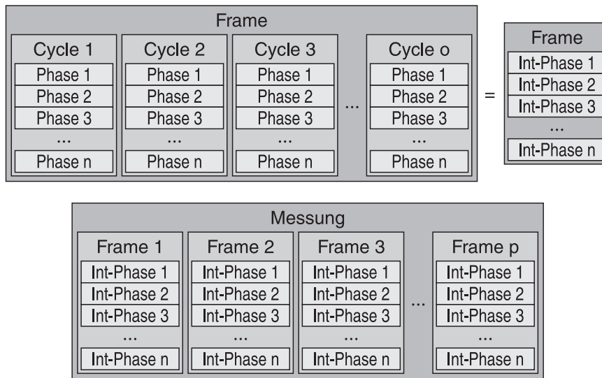
Abbildung 6.9: Die Datenstruktur einer Messung. Innerhalb eines Frames werden mehrere Zyklen mit einer immer wiederkehrenden Abfolge von Meßphasen aufintegriert. Das Frame ist die kleinste abgespeicherte Informationseinheit. Eine Messung besteht aus mehreren Frames.
