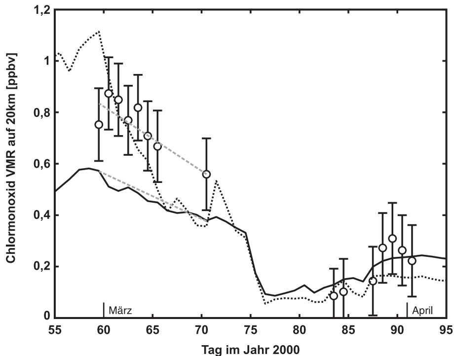
Abbildung 7.9: Die Ergebnisse des Chlormonoxid Radiometers in einer Höhe von 20 km im Vergleich zum SLIMCAT Modell. Die punktierte Linie entspricht den SLIMCAT Daten mit ihrer originalen Höhenauflösung von etwa 2 km; die durchgezogene Linie entspricht einem SLIMCAT, das auf die RAM Höhenauflösung umgerechnet wurde. Als gestrichelte, graue Linien sind zwei Tendenzlinien für die Zeit vom 29. Februar bis zum 11. März eingezeichnet.
