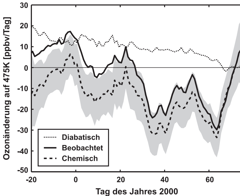
Abbildung 7.7: Die Veränderungen des Ozons auf der 475K Isentrope nach Klein et al. (2001). Gezeigt wird der vom Ozon Radiometer des RAM beobachtete Ozonverlust (dicke Linie) und die Änderung aufgrund diabatischer Abkühlung und dem sich daraus ergebenden Absinken der Luftmassen (dünne Punktlinie). Die Differenz ist der chemische Ozonverlust (dicke Punktlinie mit Fehlerbereich in grau).
