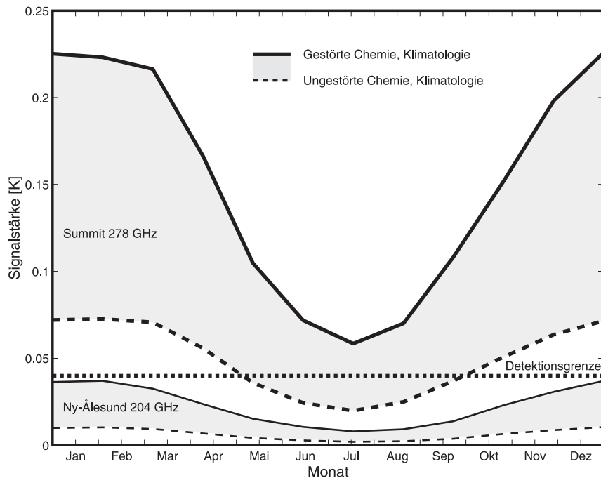
Abbildung 3.5: Ein modellierter Vergleich der Signalstärken des vorhandenen 204 GHz Radiometers in Ny-Ålesund und des geplanten 278 GHz Radiometers in Summit. Die Rechnungen wurden für einen monatlich neu bestimmten optimalen Beobachtungswinkel durchgeführt; die »Detektionsgrenze« ist nur ein geschätzter Wert. Es zeigt sich, daß in der Summit Station außer in den Sommermonaten Chlormonoxidmessungen problemlos möglich sein sollten. In Ny-Ålesund bedarf es hingegen auch in den Wintermonaten überdurchschnittlich guter Meßbedingungen.
