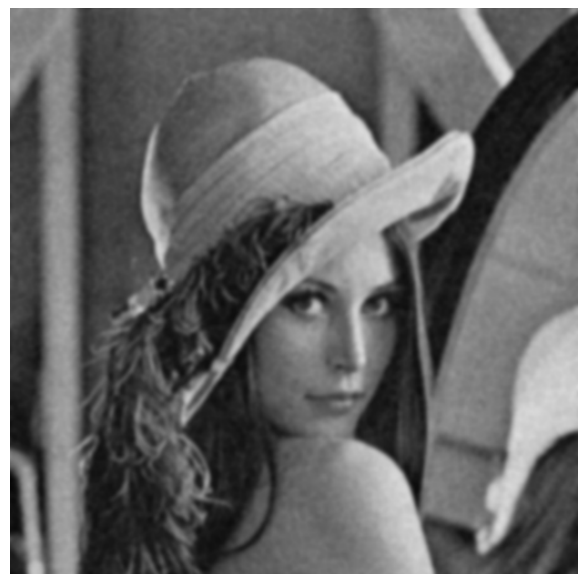
Gauß-Filter
