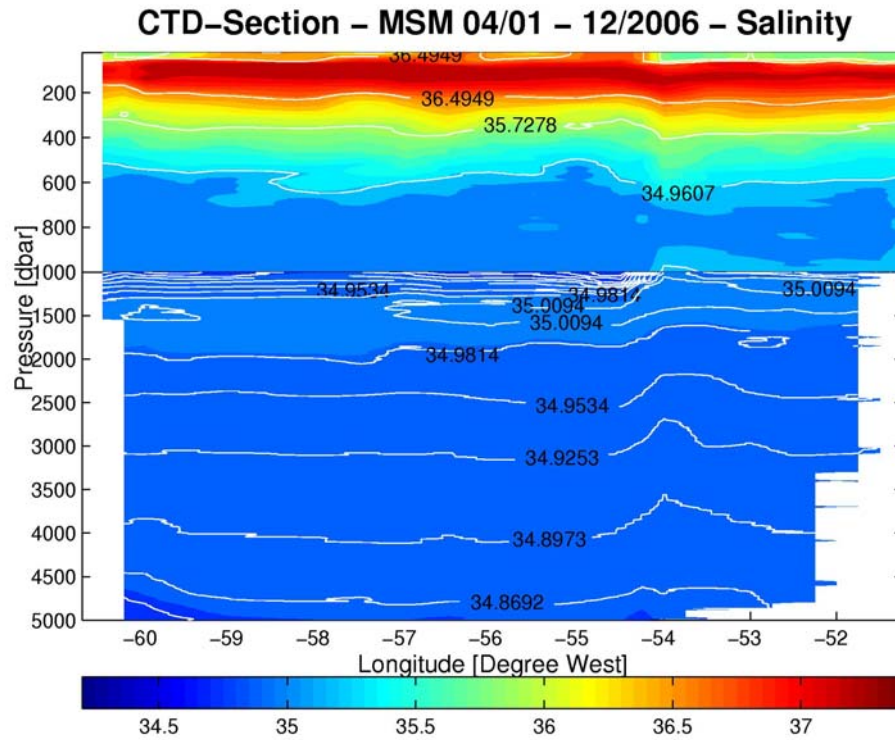
Fig. 1.2.b: MSM04/1, salinity along 16° N.
